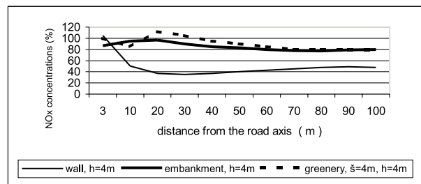
Obr. 8 Porovnanie účinku zelene, protihlukovej steny a zemného valu [3] (š - šírka, h - výška)
