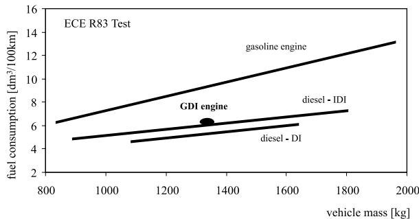
Obr. 5. Porovnanie spotreby paliva vozidiel s motormi zážihovými a vznetrovými [10]
