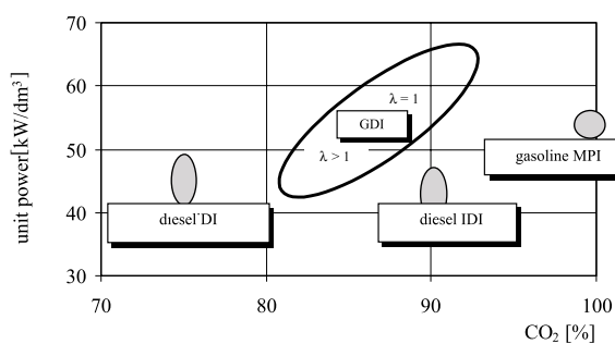
Obr. 6. Redukcie emisií CO 2 priamym vstrekaním [10]
